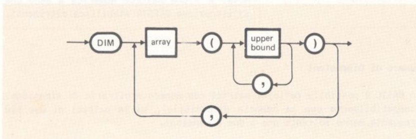
Figura 4-2 Istruzione DIM
